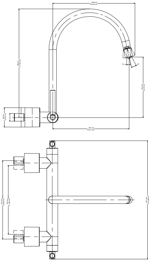
MISTURADOR P/ PIA DE COZINHA PAREDE 1/2" LINHA NOVITA - CHROME WALL-MOUNT HIGH SPOUT KITCHEN FAUCET - 1/2" - NOVITA MEZCLADOR DE PARED PICO ALTO - 1/2" - NOVITA
